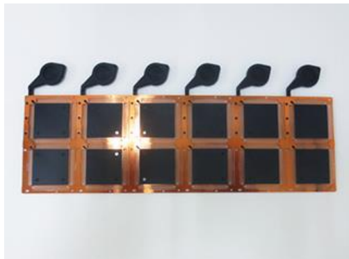
エポキシ樹脂封止後の成型物
